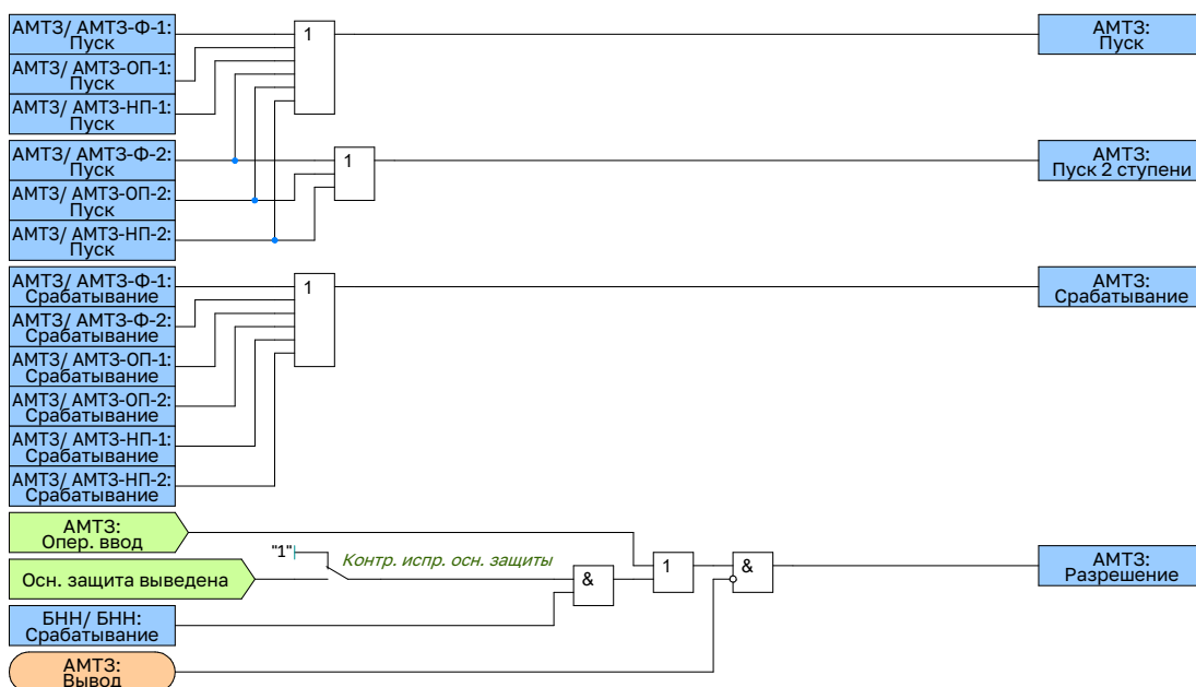
Рисунок 2.53 – Функциональная схема общей логики АМТЗ
