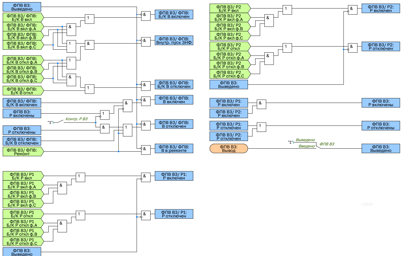
Рисунок 2.84 – Функциональная схема логики ФПВ ВЗ
