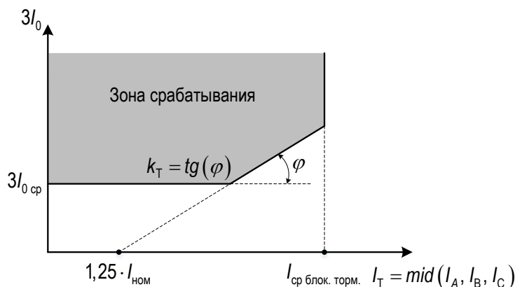
Рисунок 2.30 – Характеристика срабатывания ИО 3I 0 ООВП
